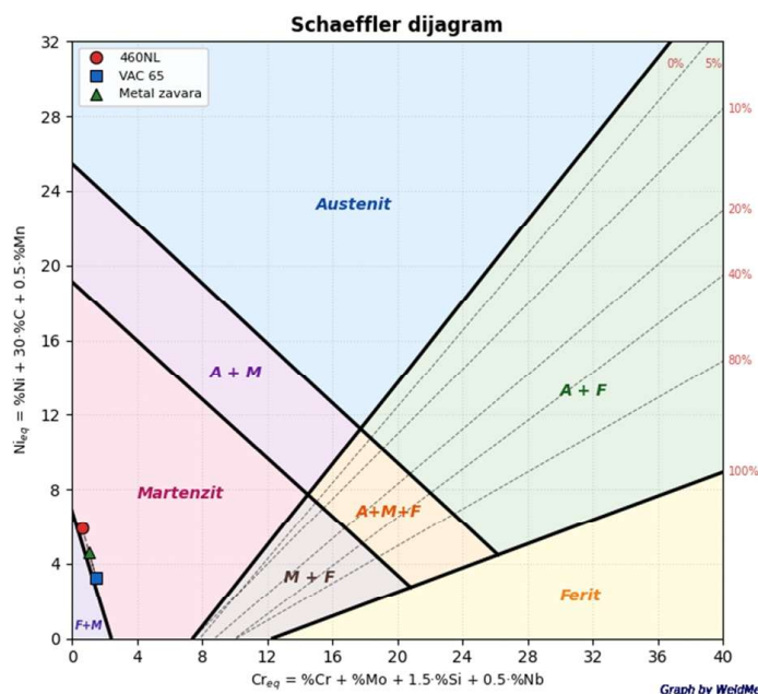
Slika 4. – Schaeffler dijagram za P 460 NL1 + VAC 65
